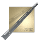
Netzhalterleiste, 0,5 m lang aus Edelstahl, 1.4301 unbehandelt, mit 4 ovalen Löchern 10 x 105 mm zum Befestigen von Perlondraht-Polypropylen-, und Polyethylen-Netzen sowie Drahtgitter
